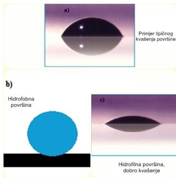
Slika 3. Vrste kvašenja površine a) primjer tipičnog kvašenja površine b) slabo kvašenje, kontaktni kut veći od 90° c) hidrofilne površine, dobro kvašenje [2]
