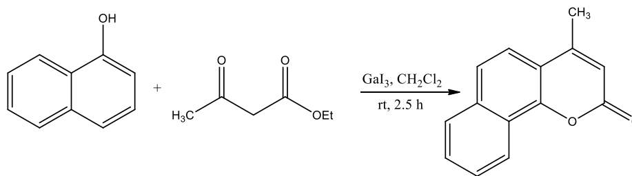
Shema 4. Modificirana Pechmannova kondenzacija uz \text{GaI}_3 kao katalizator
