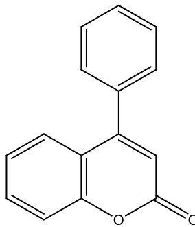
Slika 7. Opća kemijska struktura fenilkumarina
