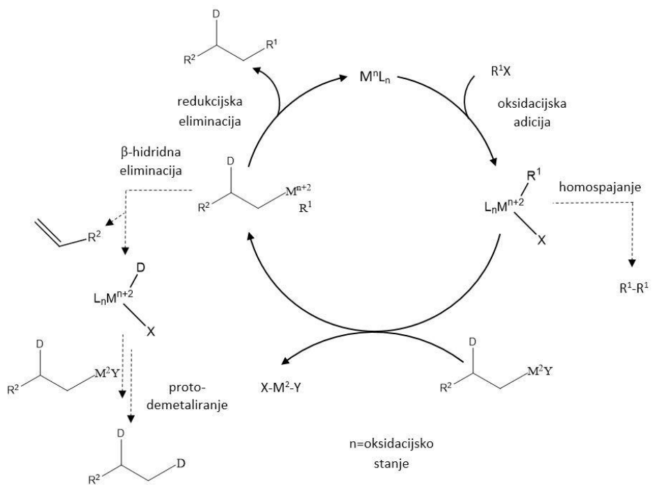
Shema 30. Mehaničke značajke organometalnih reakcija
