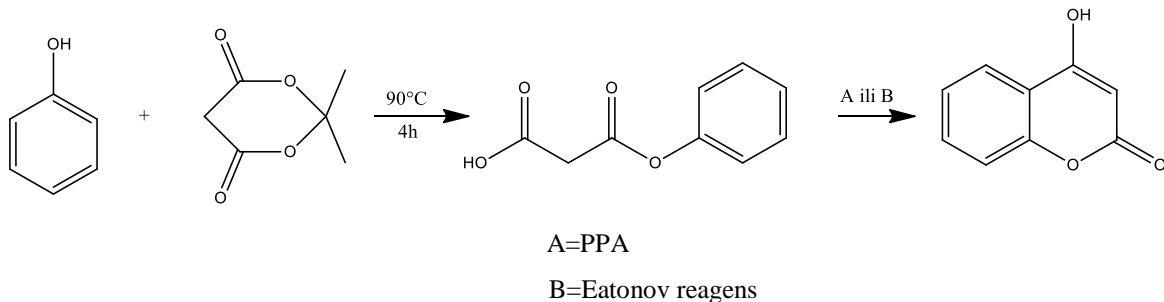
Shema 18. Sinteza 4-hidroksikumarina
