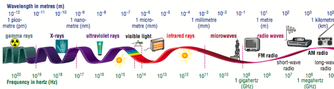
Slika 6. Elektromagnetski spektar
