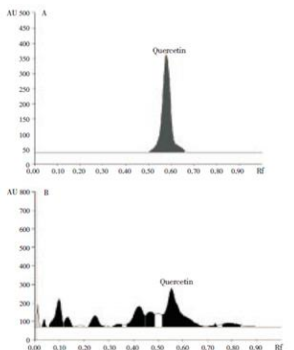
Slika 3. HPTLC denzitogram kvercetina (A) i etanolnih ekstrakcija propolisa (B)
