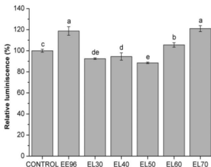
Slika 7. Energija staničnog metabolizma u kvascu S. cerevisiae tretiran sa EE96 i EL30 do EL70
