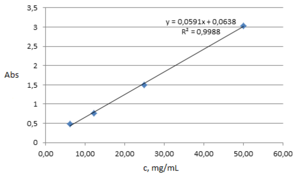
Slika 26. Grafički prikaz promjena absorbancije po promjeni koncentracije galne kiseline po mililitru uzorka (standardna krivulja)
