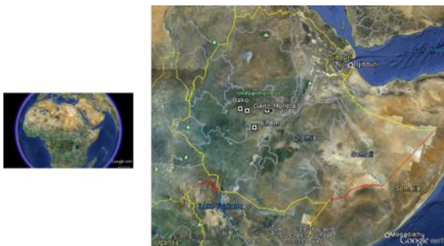
Slika 10. Područje s kojeg su prikupljeni uzorci propolisa prikazano na karti
