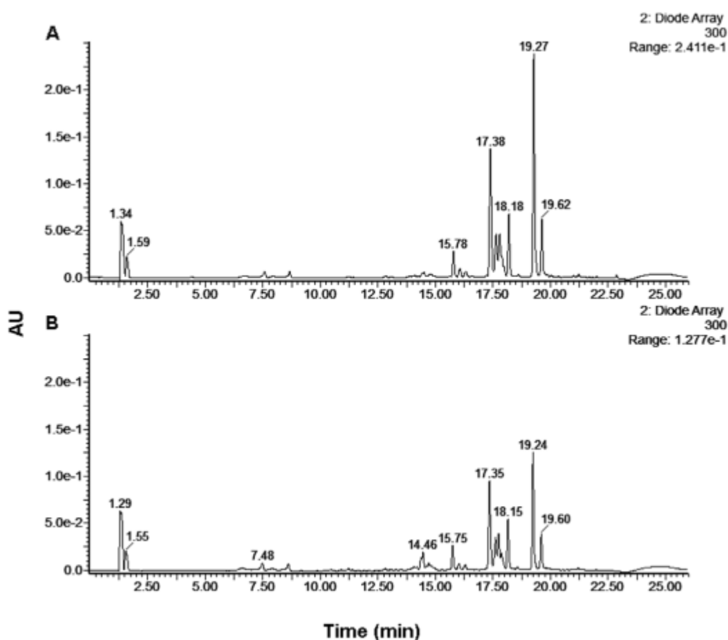
Slika 6. LC - DAD ( 300 nm ) kromatogram fenolnih spojeva u inkubacijskom mediju prije (A) i posije (B) 2h izloženosti kvasca Saccharomyces cerevisiae eluacijskoj frakciji EL70
