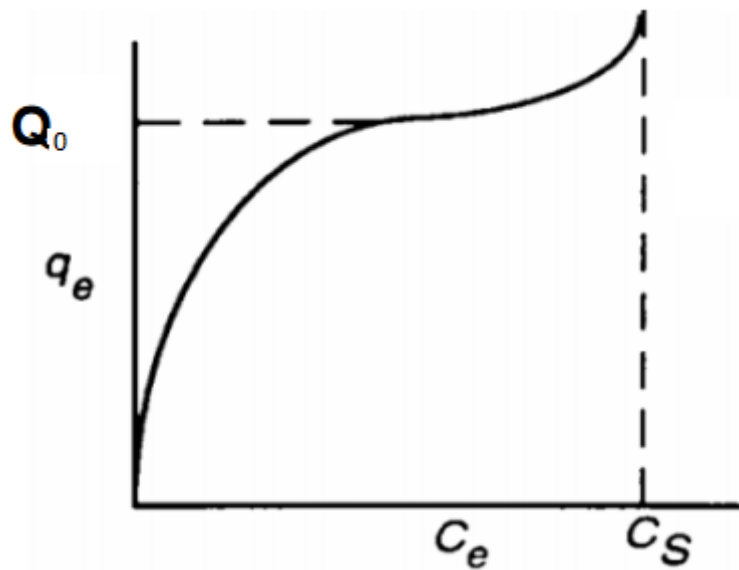
Slika 2.6. Grafički prikaz B.E.T. izoterme
