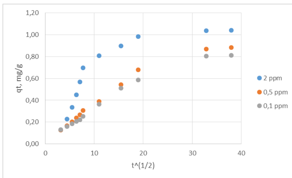
Slika 4.13. Model unutarfazne difuzije adsorpcije alendazola na sediment Sava pri koncentracijama 0,1; 0,5; 2 mg/L
