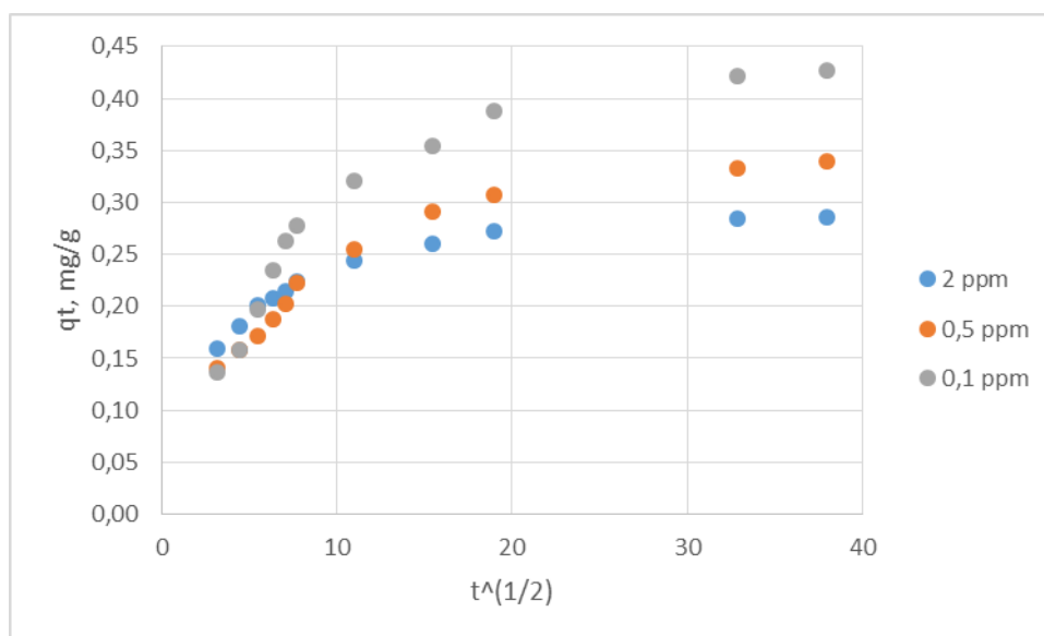
Slika 4.14. Model unutarfazne difuzije adsorpcije alendazola na tlo Topusko pri koncentracijama 0,1; 0,5; 2 mg/L
