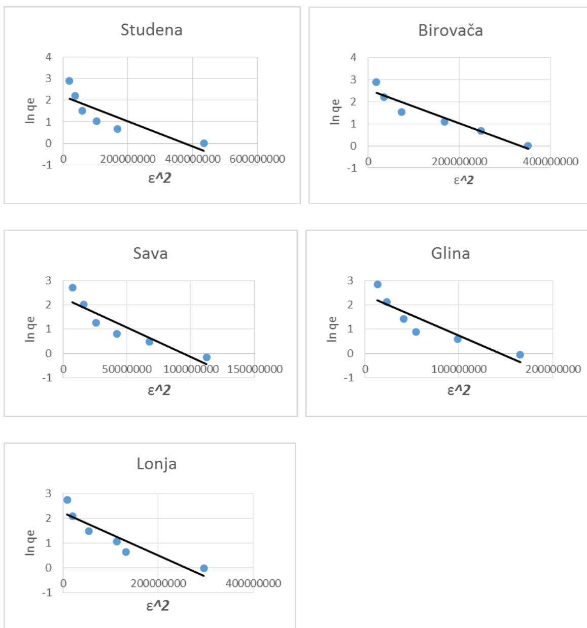
Slika 4.5. Prikaz Dubinin-Radushkevich sorpcijskih izoterma albendazola za ispitivane sedimente pri početnoj pH vrijednosti
