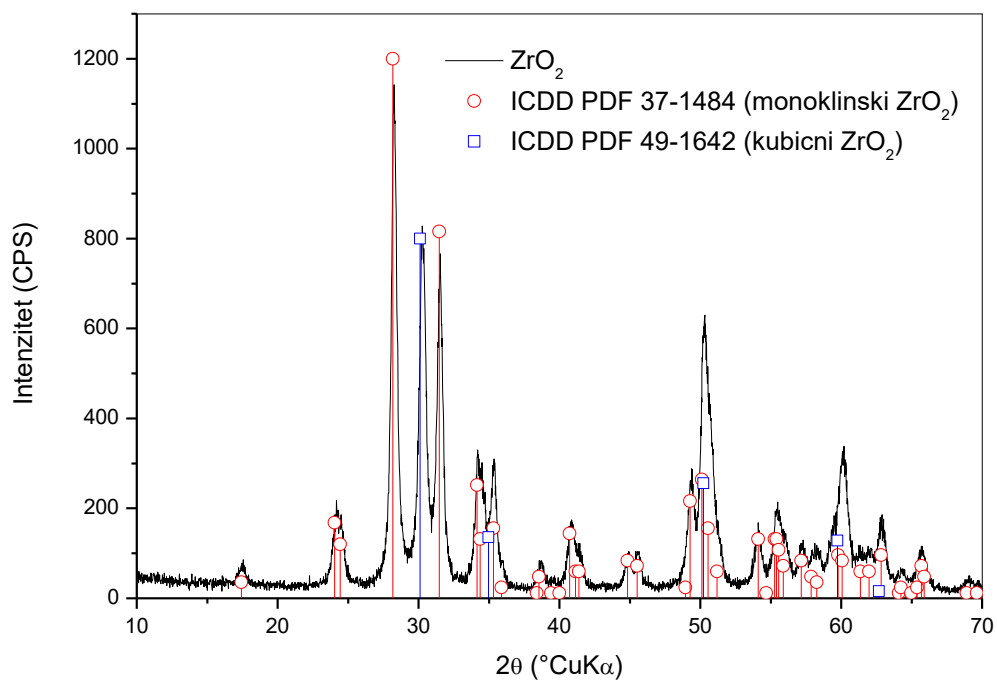
Slika 22. Difraktogram uzorka ZrO 2 .
