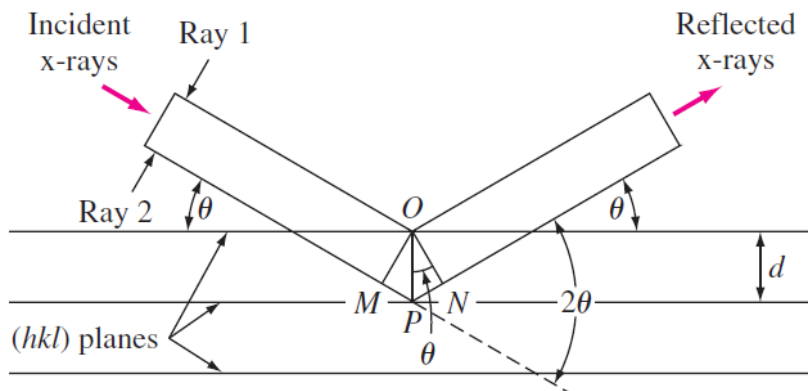
Slika 16. Difrakcija rendgenskih zraka na kristalu difrakcija na kristalu. [30]
