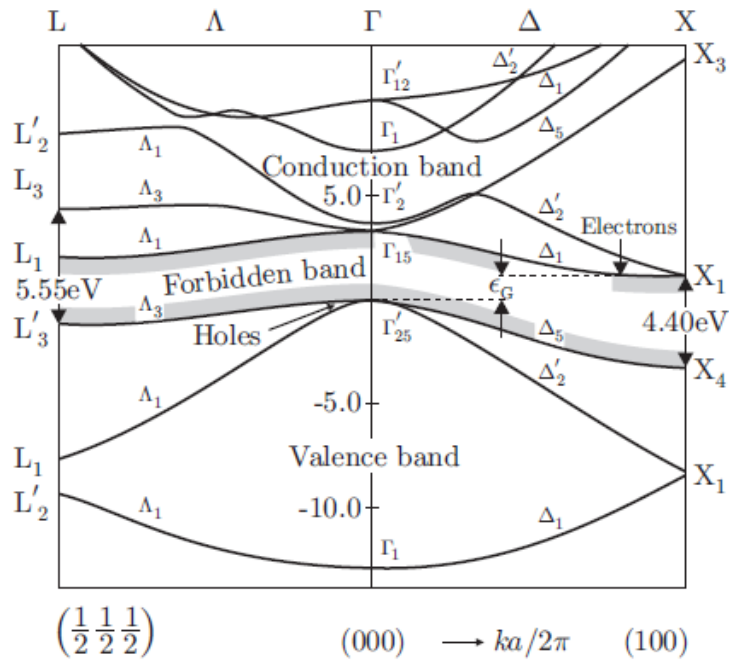
Slika 8. Struktura silicija u smjeru (100) te (111). Osjenčano područje prikazuje najniži dio (nezaposjednut pri T = 0 K) vodljive vrpce te najvišu dio (zaposjednut pri T=0 K) valentne vrpce sa zabranjenom zonom između njih. [13]
