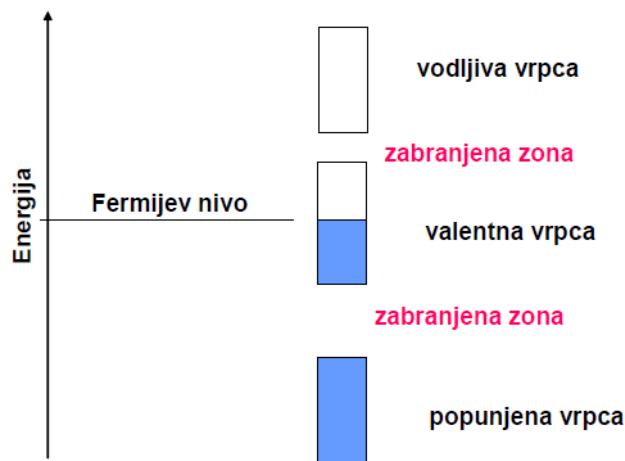
Slika 1. Shematski prikaz energijskih vrpca u čvrstom tijelu ( metalu). [3]
