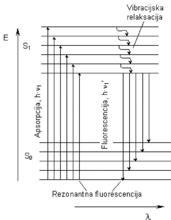
Slika 6. Dijagram fluorescencije
