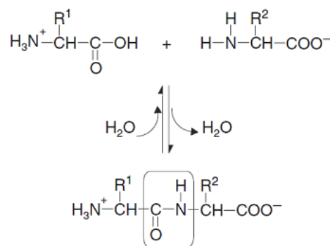
Slika 2.1. Formacija peptidne veze između dvije susjedne α-amino kiseline
