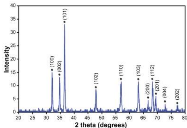
Slika 7. Difraktogram cinkovog oksida [14]
