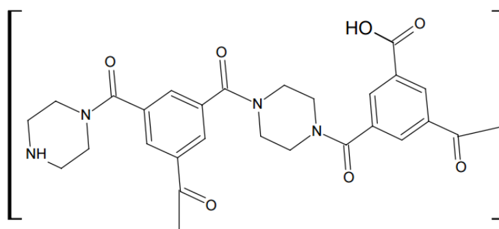
Slika 10. Približna struktura poliaromatskog poliamida polipiperazina zasnovanog na trimezol kloridu i piperazinu
