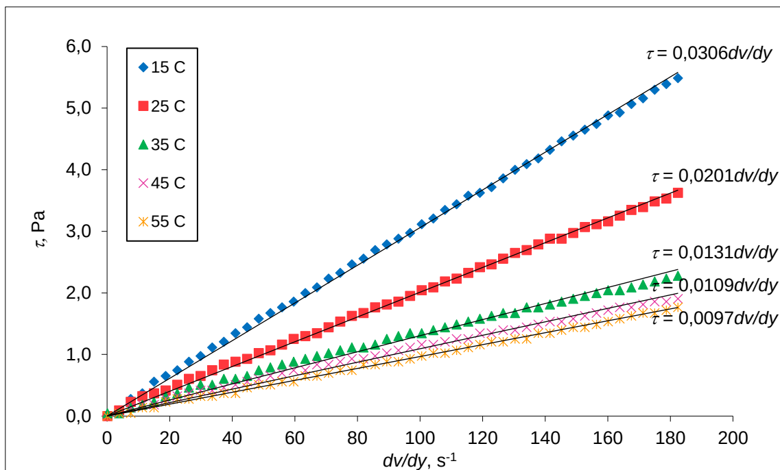
Slika 28. Dijagram ovisnosti promjene smičnog naprezanja, \tau s promjenom smične brzine, dv/dy za nanosuspenziju ChCl:Ma 1:1 30% H_2O s Al_2O_3 nanočesticama 0,3 vol% pri različitim temperaturama.
