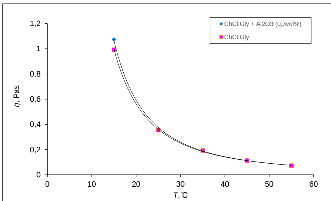
Slika 25. Dijagram prikazuje promjenu viskoznosti nanosuspencije ChCl:Gly 1:2 0% H_2O + Al_2O_3 (0,3vol%) s temperaturom.
