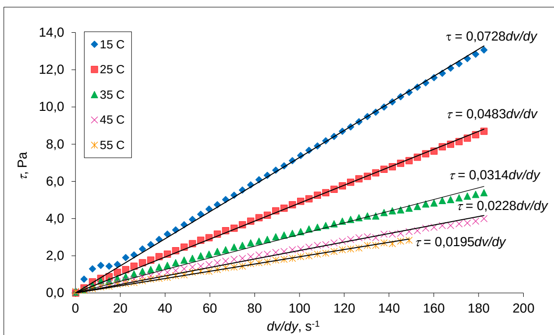
Slika 22. Dijagram ovisnosti promjene smičnog naprezanja, \tau s promjenom smične brzine, dv/dy za nanosuspenziju ChCl:EG 1:2,5 0% H_2O s Al_2O_3 nanočesticama 0,3 vol% pri različitim temperaturama.
