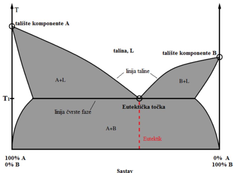
Slika 5. Fazni dijagram za zamišljenu smjesu dviju komponenata 19
