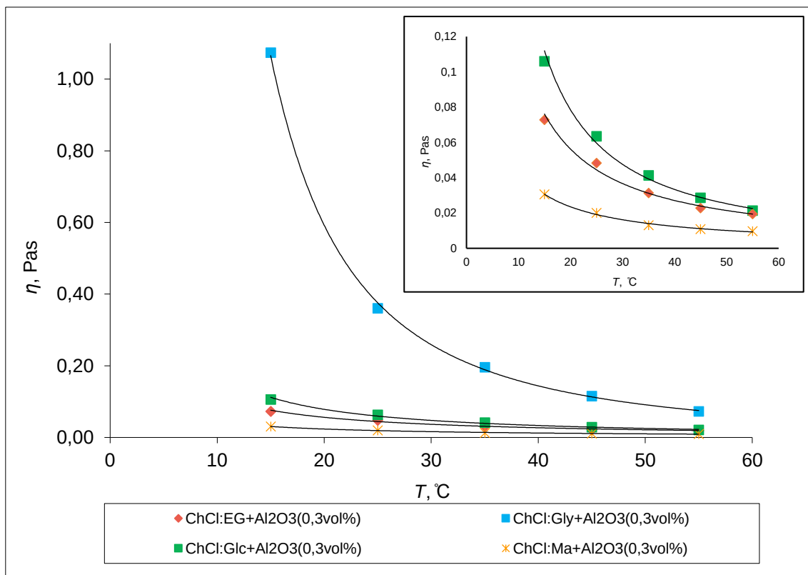
Slika 30. Dijagram prikazuje usporedbu viskoznosti s temperaturom za pripremljene nanosuspenzije s Al 2 O 3 nanočesticama volumnog udjela 0,3%.
