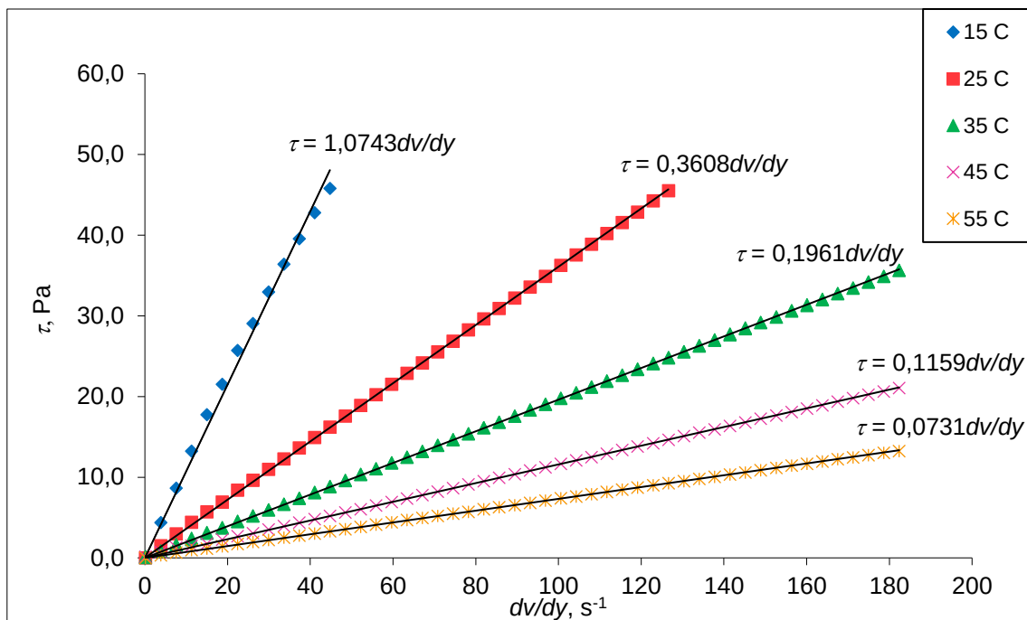
Slika 24. Dijagram ovisnosti promjene smičnog naprezanja, \tau s promjenom smične brzine, dv/dy za nanosuspenciju ChCl:Gly 1:2 0% H_2O s Al_2O_3 nanočesticama 0,3 vol% pri različitim temperaturama.
