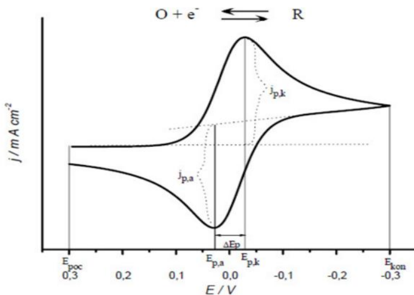
Slika 2.15. Ciklički voltamogram reverzibilnih elektrodskih procesa
