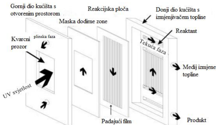
Slika 15. Mikroreaktor s padajućim filmom [7]
