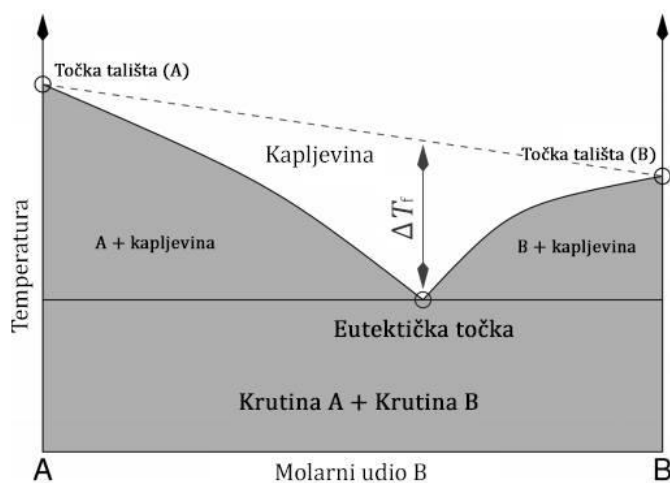
Slika 7. Fazni dijagram dvokomponentne eutektičke smjese 7
