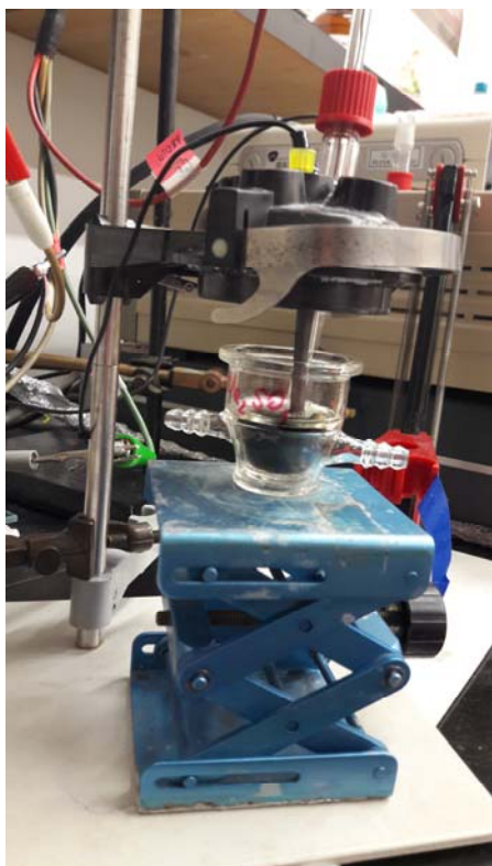
Slika 3.2. Elektrokemijska ćelija s a) dvoelektrodnim sustavom korištena za elektrokemijsko raslojavanje grafita i b) troelektrodnim sustavom korištena tijekom snimanja cikličkih voltamograma
