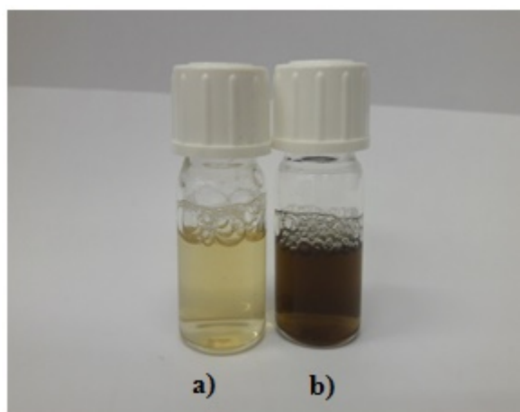
Slika 4.19. Otopine dobivene nakon polarizacije a) priređene elektrode i b) grafitnog štapića u 0,1 mol dm -3 SDS pri 3,2 V
