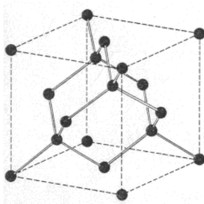
Slika 2.1. Struktura dijamanta.
