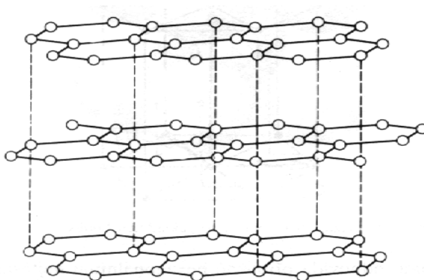
Slika 2.2. Struktura grafita.
