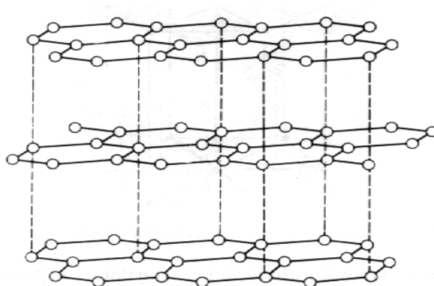
Slika 2.2. Struktura grafita.
