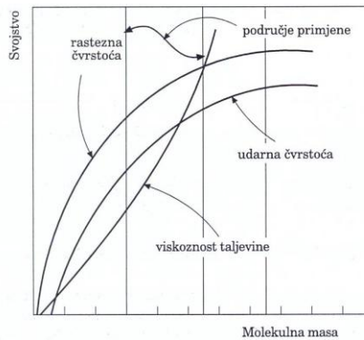
Slika 1. Utjecaj molekularne mase na neka mehanička svojstva plastomera
