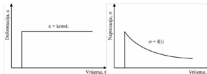
Slika 12. Relaksacija naprezanja
