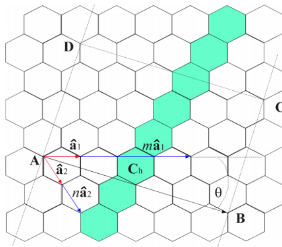
Slika 16. Šesterokutna rešetka ugljikovih atoma: konstrukcija nanocjevčice ( m, n ) = (4, 2)
