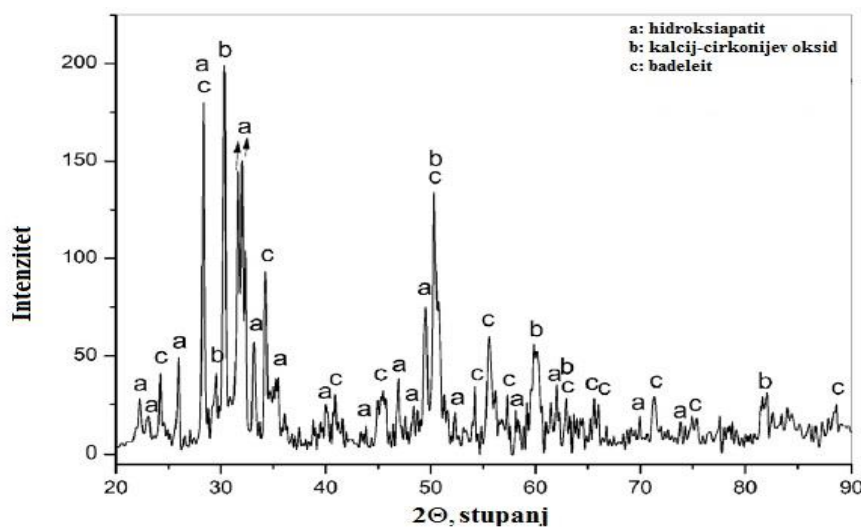
Slika 6. XRD uzorka cirkonija obloženog hidroksiapatitom
