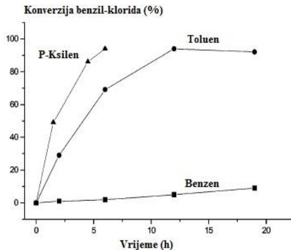
Slika 11. Ovisnost konverzije benzil-klorida o vremenu
