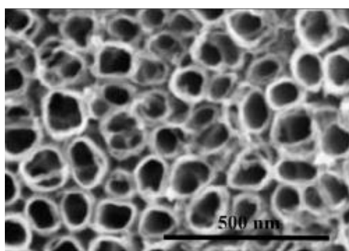
Slika 13. SEM prikaz uredno poredanih nanocjevčica \text{TiO}_2
