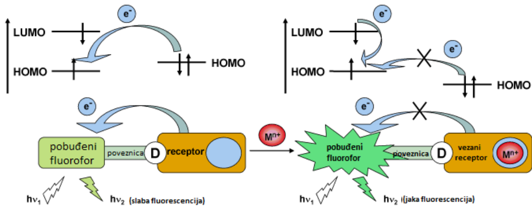
Slika 14. PET mehanizam [36]
