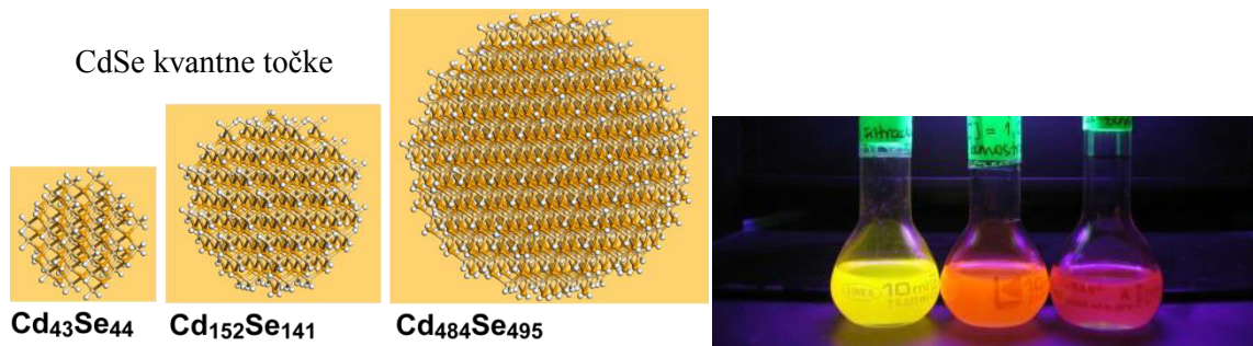
Slika 6. CdSe kvantne točke - strukturalni prikaz (lijevo), trend porasta valne duljine fluorescencije pod UV-zračenjem s porastom veličine čestica (desno)
