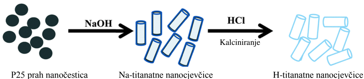
Slika 12. Sažeti shematski prikaz hidrotermalne sinteze Na-oblika titanatnih nanocjevčica i prevođenja u H-oblik titanatnih nanocjevčica
