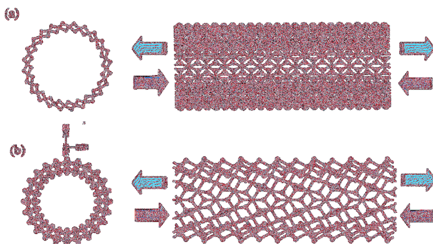
Slika 11. Dvije krajnje moguće strukture titanatnih nanocjevčica - „naslonjač“ (gore) i „cikcak“ (dolje)
