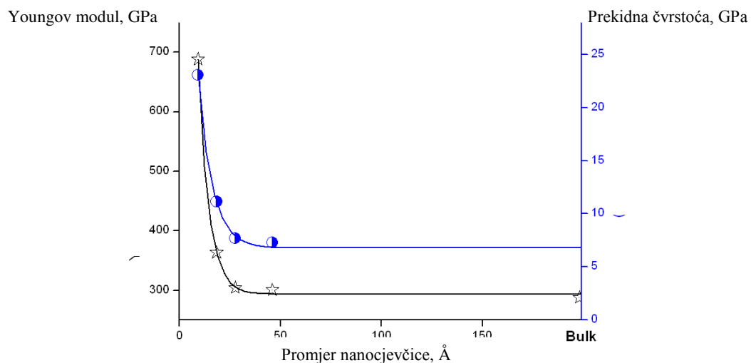
Slika 14. Grafički prikazi Youngovog modula elastičnosti i prekidne čvrstoće na vlak za \text{TiO}_2 nanocjevčice, u odnosu na promjer cjevčice
