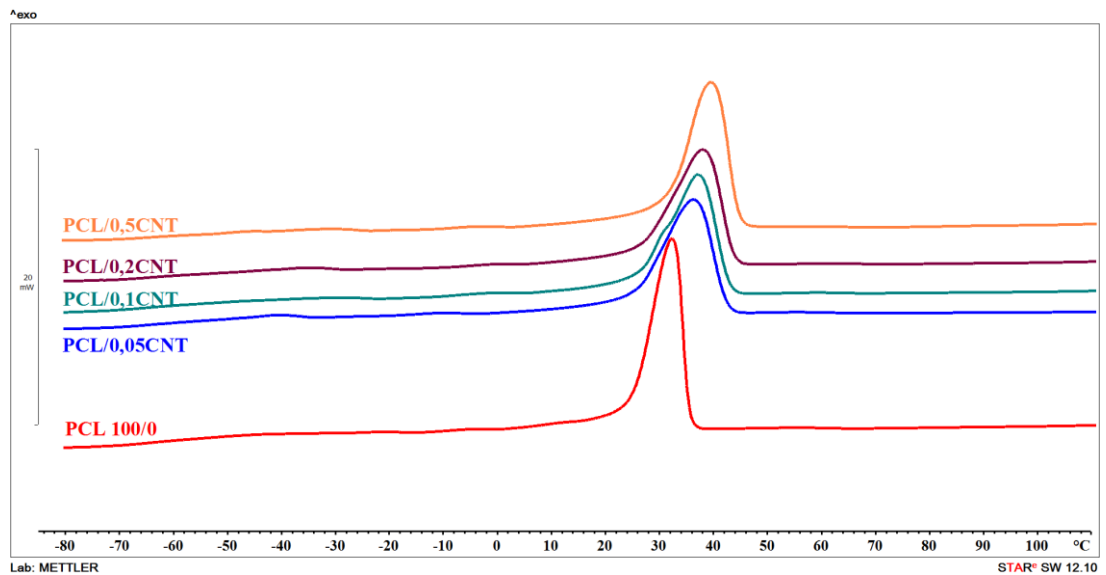
Slika 22. DSC krivulje zagrijavanja i hlađenja za PCL i PCL/CNT nanokompozite dobivenih umiješavanjem u Brabender gnjetilici.
