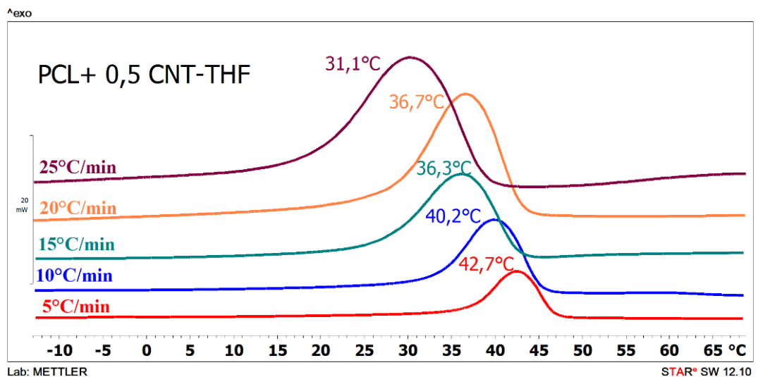
Slika 25. Egzotermi kristalizacije dobiveni na različitim brzinama hlađenja za PCL i PCL+0,5mas% CNT nanokompozit dobivenog umiješavanjem u Brabender gnjetilici i THF-
