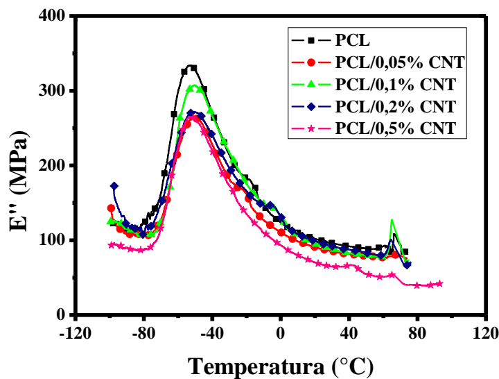
Slika 27. Krivulja modula gubitka u ovisnosti o temperaturi za PCL i PCL/CNT nanokompozite pripravljene u a) Brabender gnjetilici i b) THF-u.
