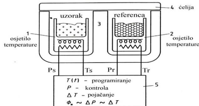
Slika 10. Kompenzacijski diferencijalni pretražni kalorimetar.
