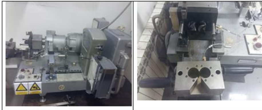
Slika 13. Brabender gnjetilica.
