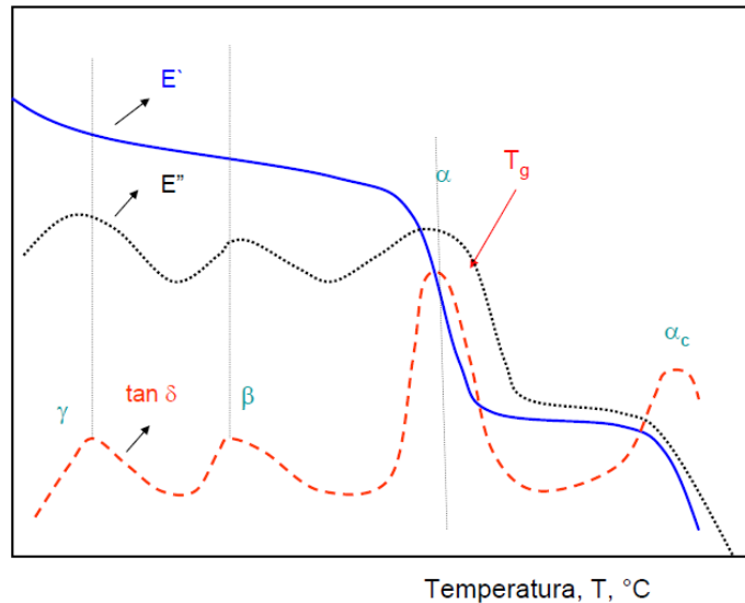
Slika 12. DMA spektr.
