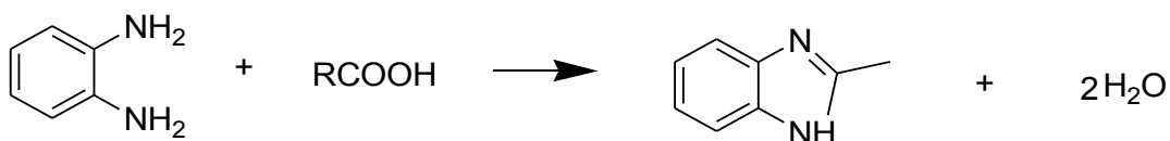
Slika 7. Reakcija dobivanja benzimidazola iz o -fenilendiamina
