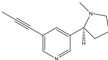
Slika 45. Struktura altiniclina
