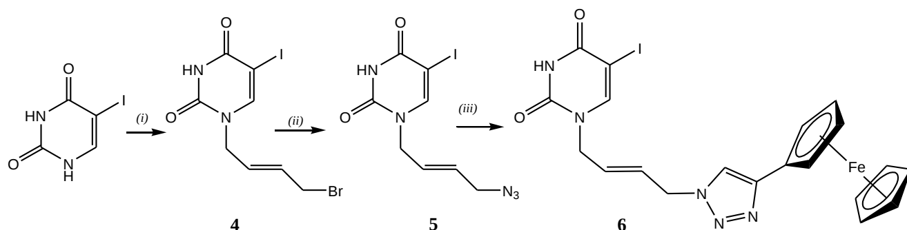
Shema 2.
