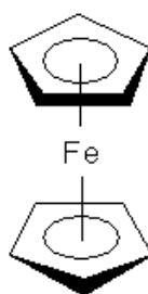
Slika 30. Struktura ferocena
