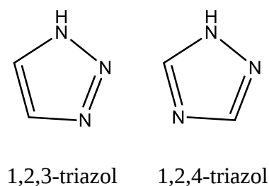
Slika 39. Izomeri triazola
