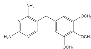
trimetoprim
