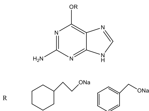
Slika 27.. O-6-alkilgvanin derivati
