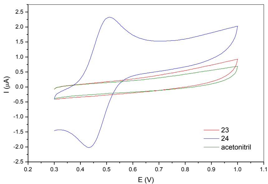
Slika 23. Ciklički voltamogram spojeva 23 i 24 u 0,1 mol dm -3 LiBF 4 u acetonitrilu
