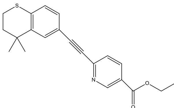
Slika 44. Struktura tazarotena.
