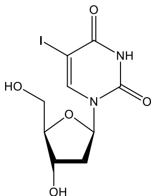
jodoksouridin
