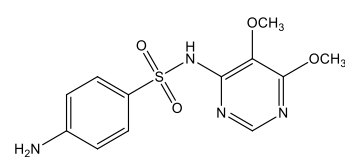
sulfadoksin
