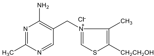
Slika 6. Tiamin
