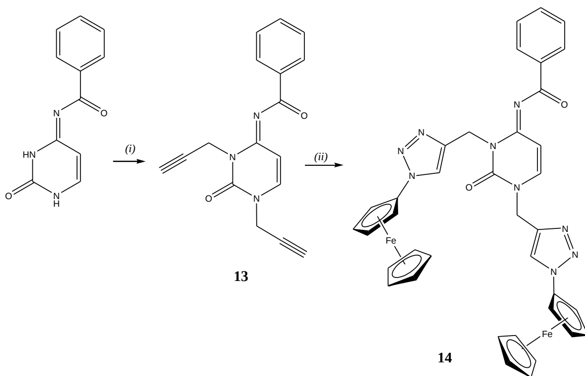
Shema 4.
