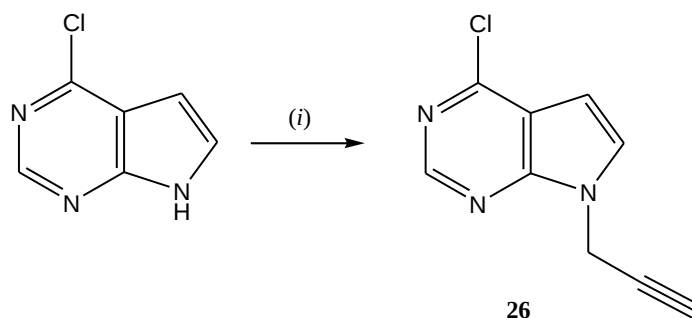
Shema 8.
