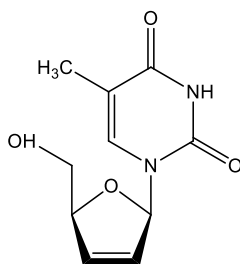
stavudin
