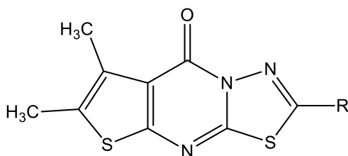
Slika 21. Supstituirani (1,3,4)-tiadiazolotieno[3,2- e ]primidin5(4 H )-eni
