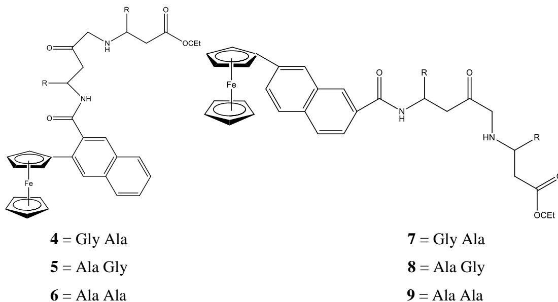
Slika 32. Derivati N-(feroceni)-naftalena
