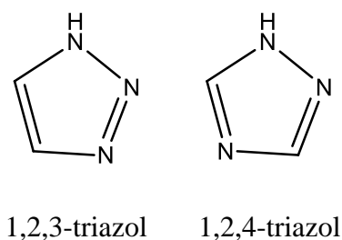
Slika 39. Izomeri triazola
