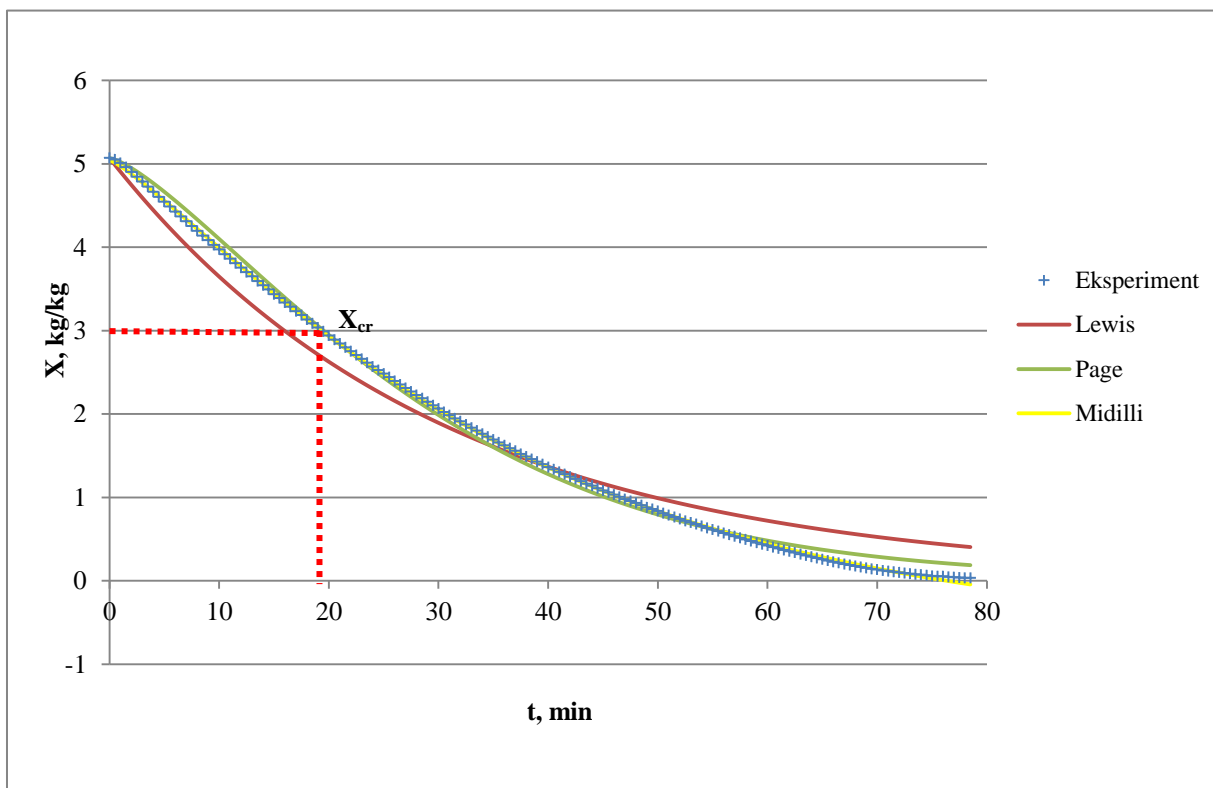
Slika 86. Grafički prikaz promjene sadržaja vlage uzorka poriluka s vremenom pri 80\text{ }^{\circ}\text{C} te primjenjivost Lewis -ovog, Page -ovog i Midilli-Kucuk -ovog modela
