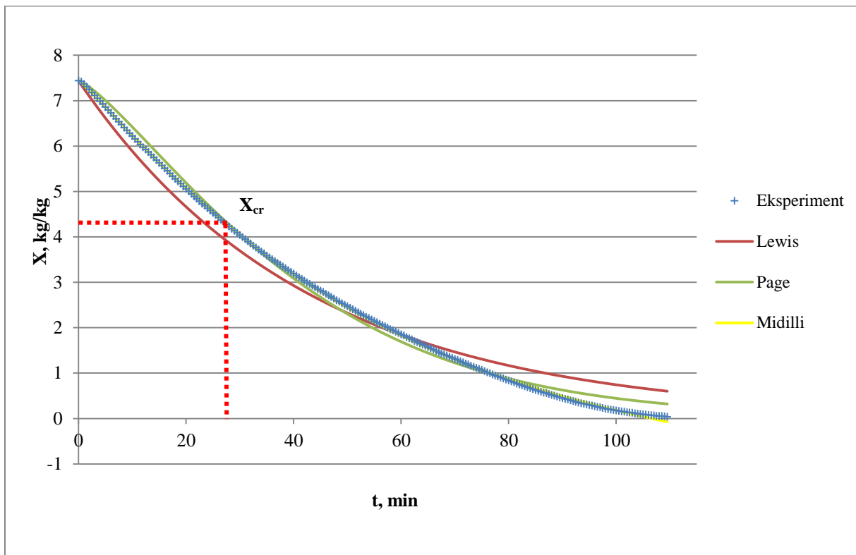
Slika 85. Grafički prikaz promjene sadržaja vlage uzorka poriluka s vremenom pri 70\text{ }^{\circ}\text{C} te primjenjivost Lewis -ovog, Page -ovog i Midilli-Kucuk -ovog modela
