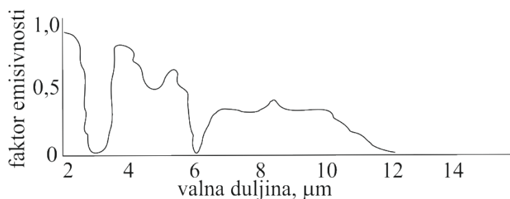
Slika 8. Apсорpcijski spektar vode
