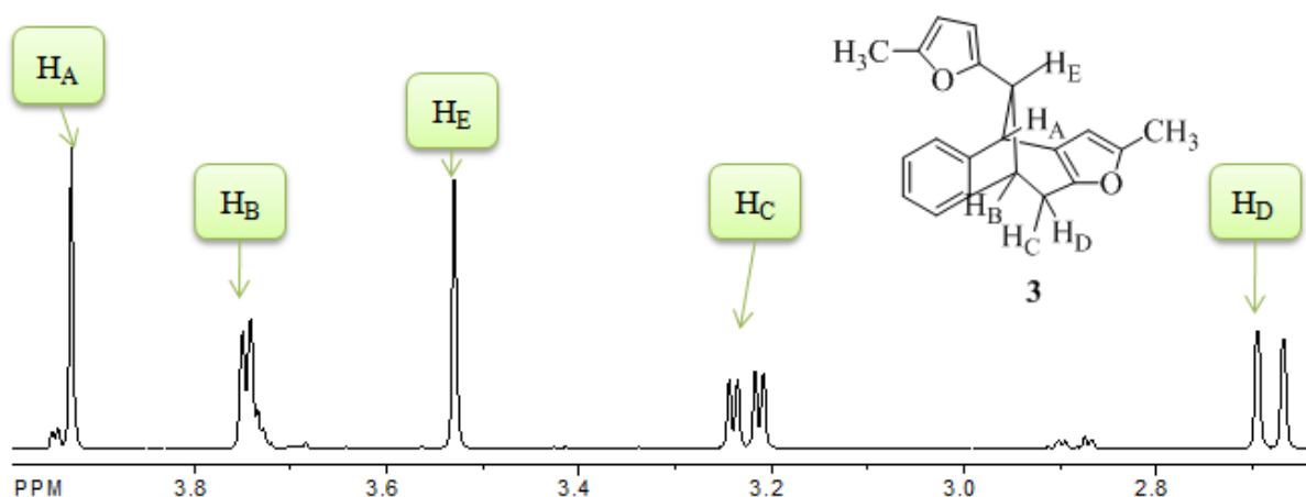
Slika 7. Alifatski dio ^1\text{H} NMR spektra fotoprodukta 3
