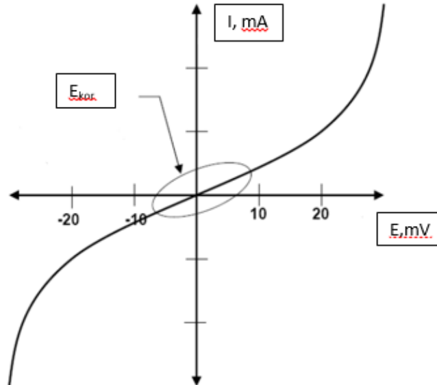
Slika 3.4. Prikaz ovisnosti struje o potencijalu u blizini korozijskog potencijala. [4]
