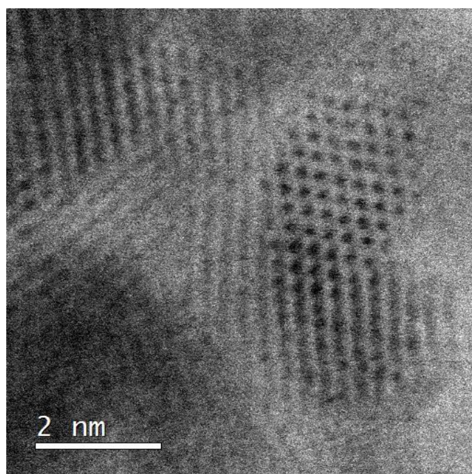
Slika 22. TEM mikrografija uzorka CeO 2 dopiranog s bakrom.
