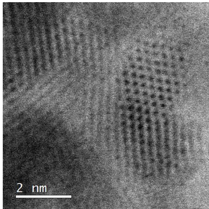
Slika 22. TEM mikrografija uzorka \text{CeO}_2 dopiranog s bakrom.
