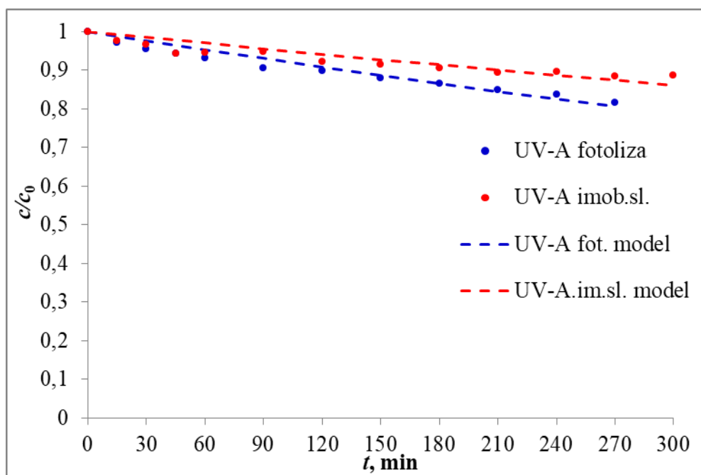
Slika 4.7. Utjecaj UV-A zračenja na fotolizu i izvedbu s imobiliziranim slojem ( c_{F0} = 12,5 mg/L, T = 30 °C, Q_R = 300 mL/min)
