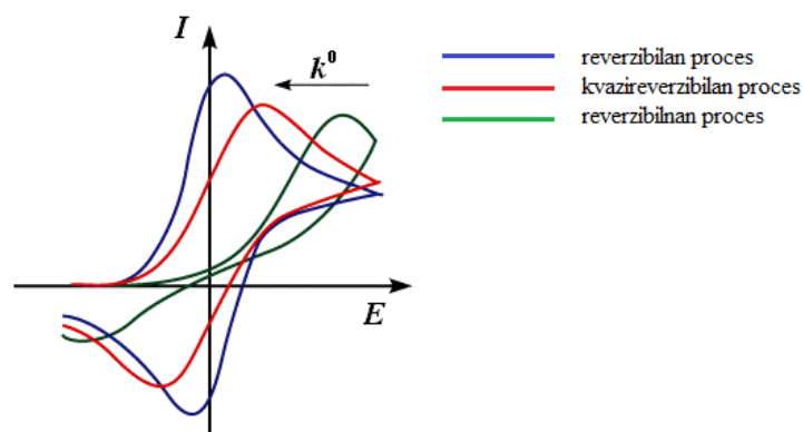
Slika 2.22. Ciklički voltamogram redukcije/oksidacije (R/O) različitih reverzibilnosti procesa koji se zbivaju u sustavu
