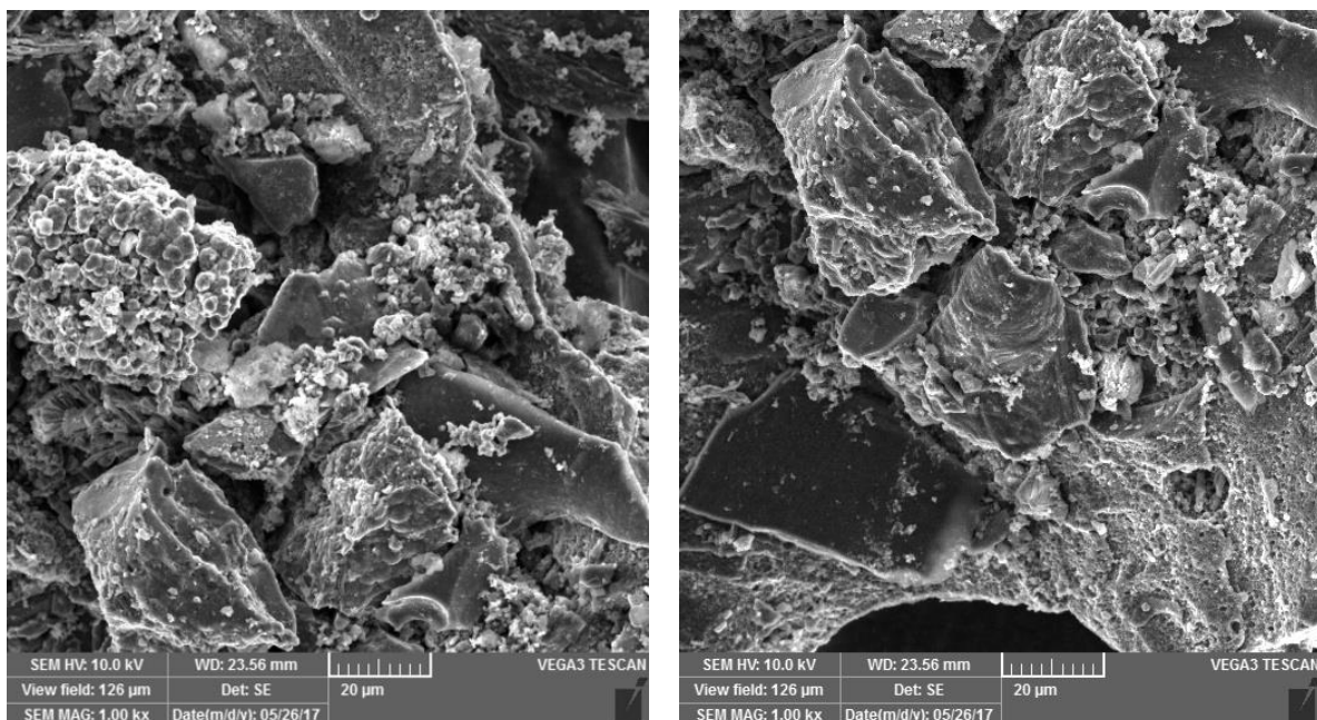
Slika 43. SEM snimak MET koksa pri uvećanju 1000x (20 µm)
