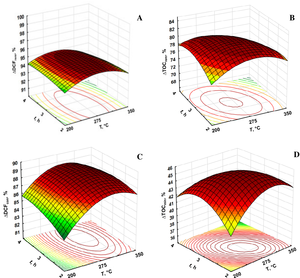
Slika 17. Odzivne površine istraženih učinaka temperature i trajanja toplinske reaktivacije prema punom faktorskom planu za uklanjanje A) DCF-a i B) TOC-a; te konverziju C) DCF-a te D) TOC-a (mineralizacija).
