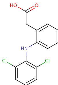
Slika 2. Molekulska struktura diklofenaka (DCF).
