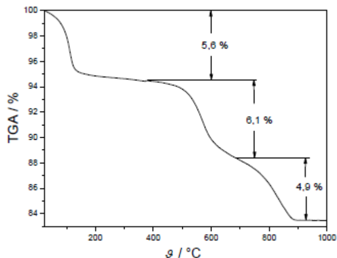
Slika 8. Primjer TGA krivulje s tri stupnja gubitka mase 22
