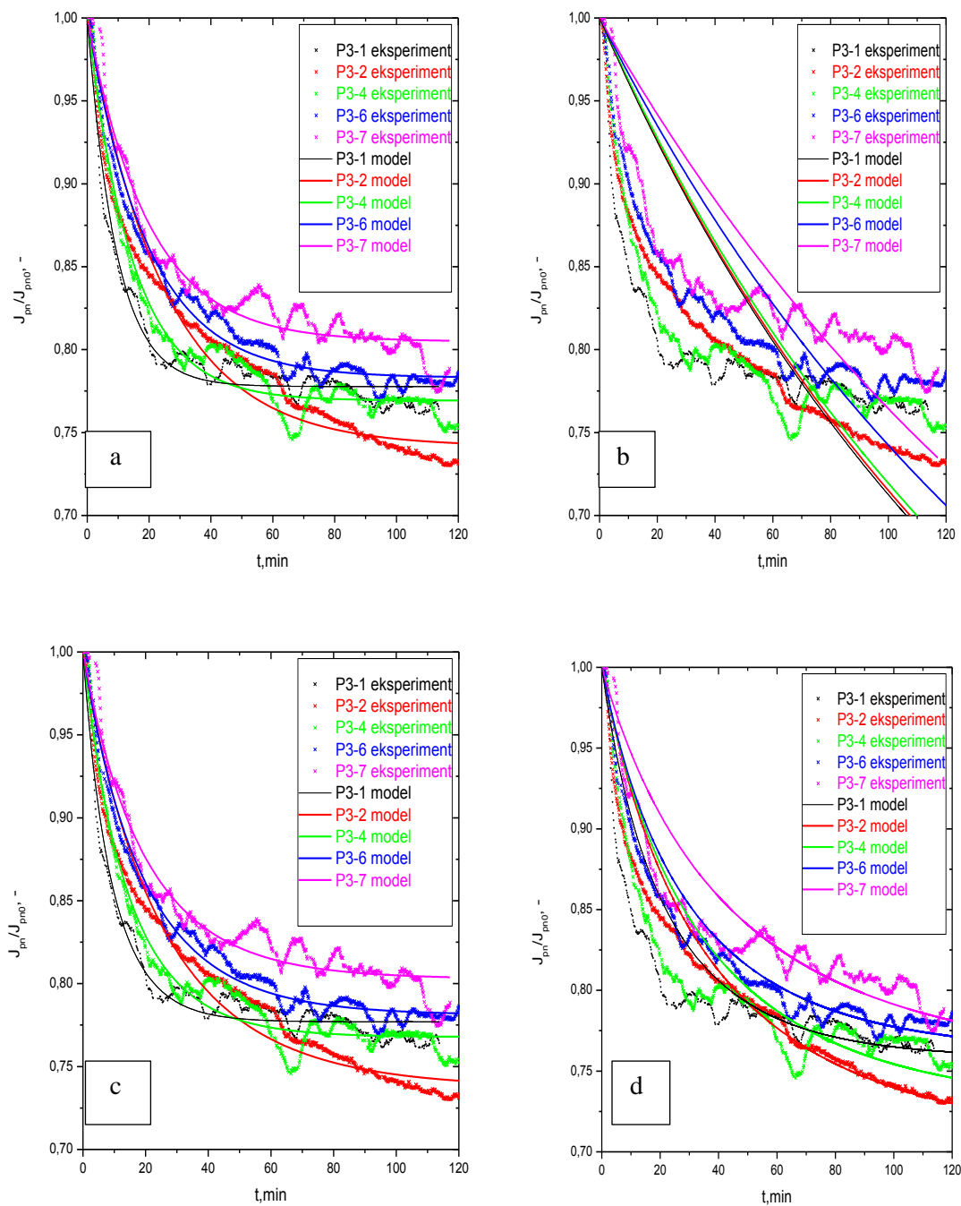
Slika 4.8. Promjena fluksa permeata NF90 membrane dobivne s otopinom PEG 1 500 različitih koncentracija prema modelu modificiranom za ukriženo strujanje: (a) CB, (b) IPB, (c) PPB i (d) CF.
