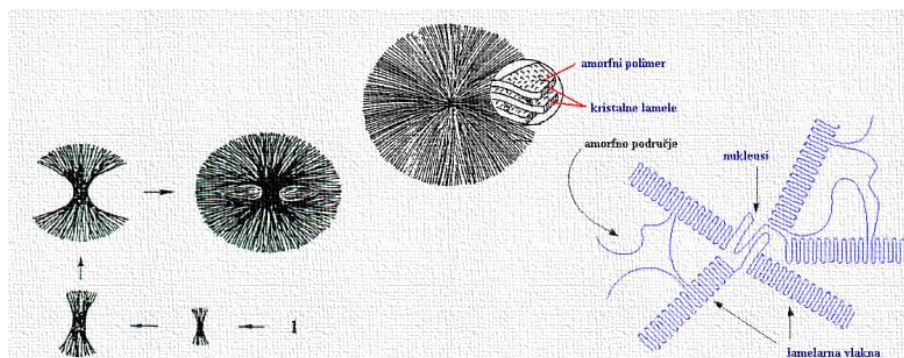
Slika 3. Rast kristala iz nukleusa, potom lamela do sferolita
