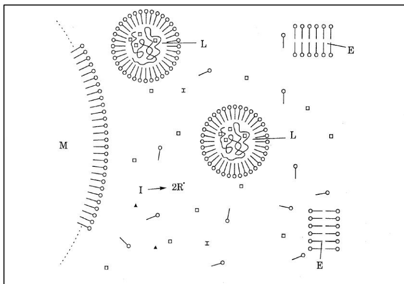
Slika 2. Shema emulzijske polimerizacije: kapljice monomera (M) i molekule monomera ( \square ), micela emulgatora (E), čestice lateksa (L), inicijator (I) i slobodni radikali ( R\cdot ) 6
