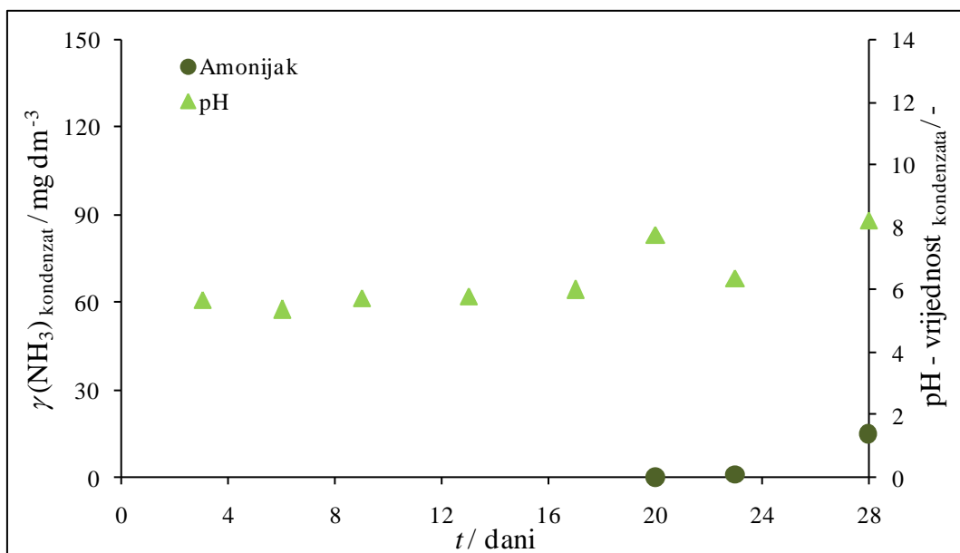
Slika 4.23. Promjena koncentracije \text{NH}_3 i pH-vrijednosti u kondenzatu tijekom 28 dana u pokusu P2.
