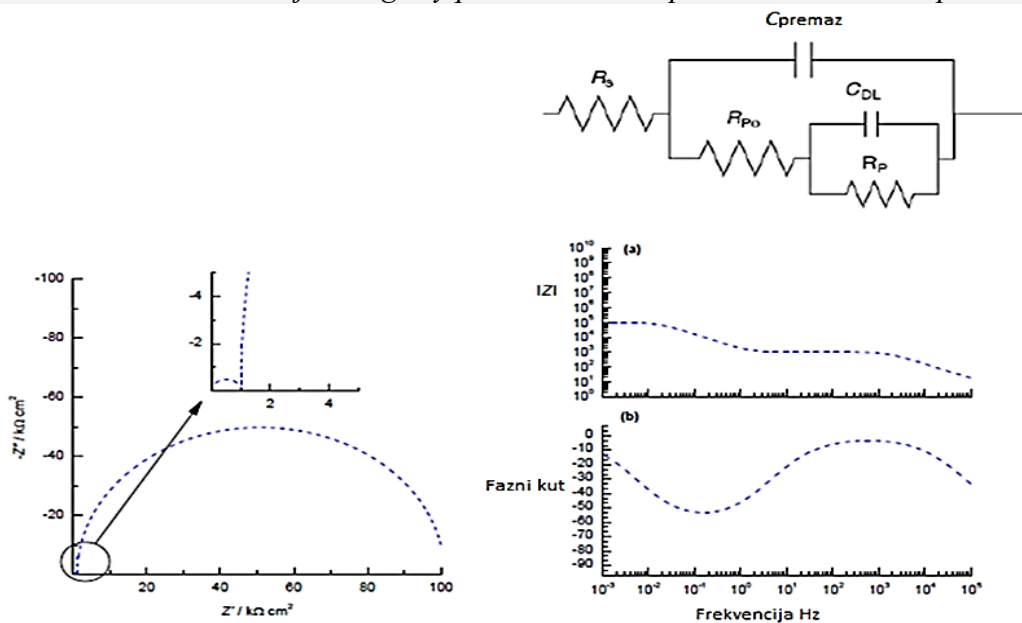
Slika 13. Ekvivalentni strujni krug, Nyquistov i Bodeov prikaz za oštećeni premaz [35]
