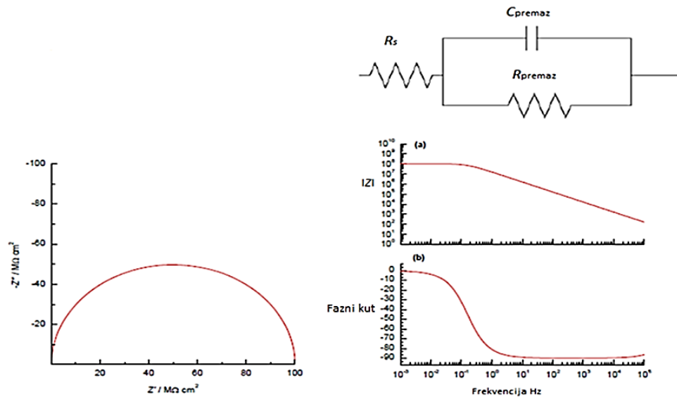
Slika 12. Ekvivalentni strujni krug, Nyquistov i Bodeov prikaz za neoštećeni premaz [35]
