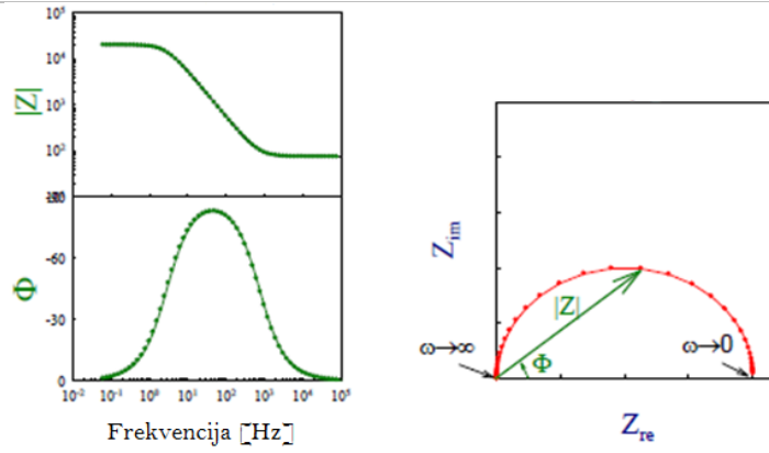
Slika 11. Općeniti prikaz Bodeovog (lijevo) i Nyquistovog (desno) dijagrama [35]
