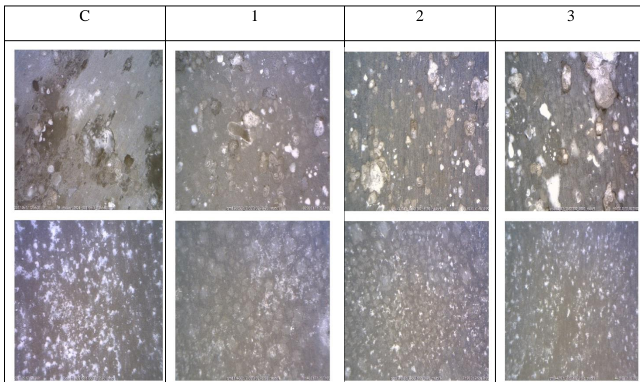
Tablica 9. Fotografije pločica nakon 7 dana izlaganja 3,5 % otopini NaCl-a s različitim koncentracijama otopljenog VCI (1,2,3) i čistoj 3,5 % otopini NaCl-a (C) snimljene svjetlosnim mikroskopom na dijelu pločica uronjenom u elektrolit (dolje) i na dijelu pločica iznad elektrolita (gore).
