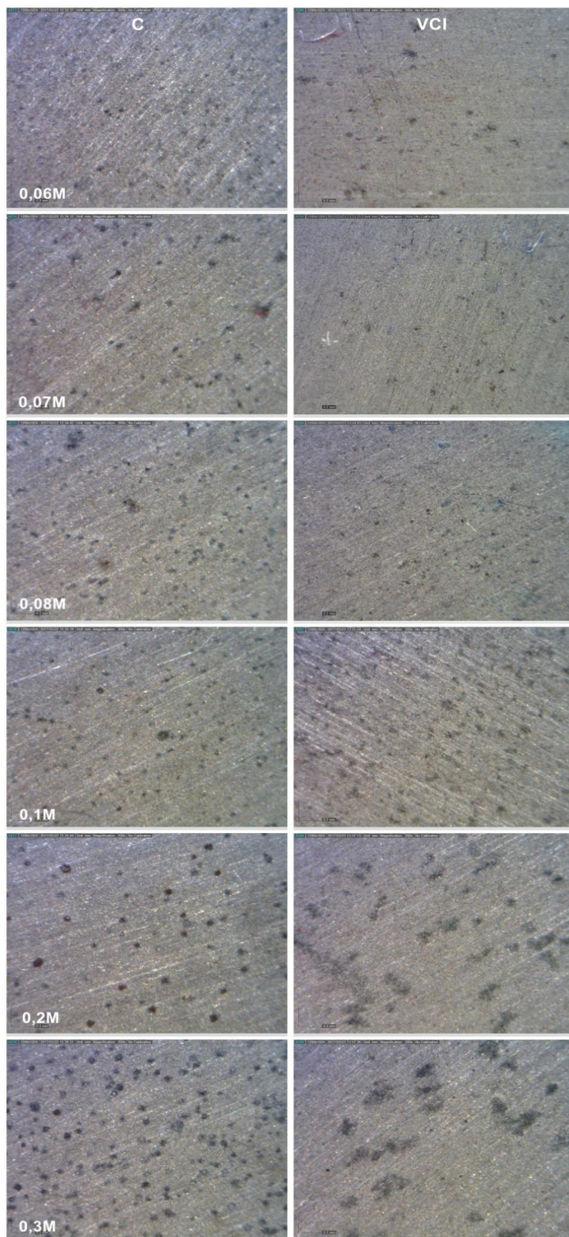
Slika 22. Neinhibirane (C) i inhibirane (VCI) testne površine nakon izlaganja bakrovim ionima snimljene svjetlosnim mikroskopom pod povećanjem 200 x.
