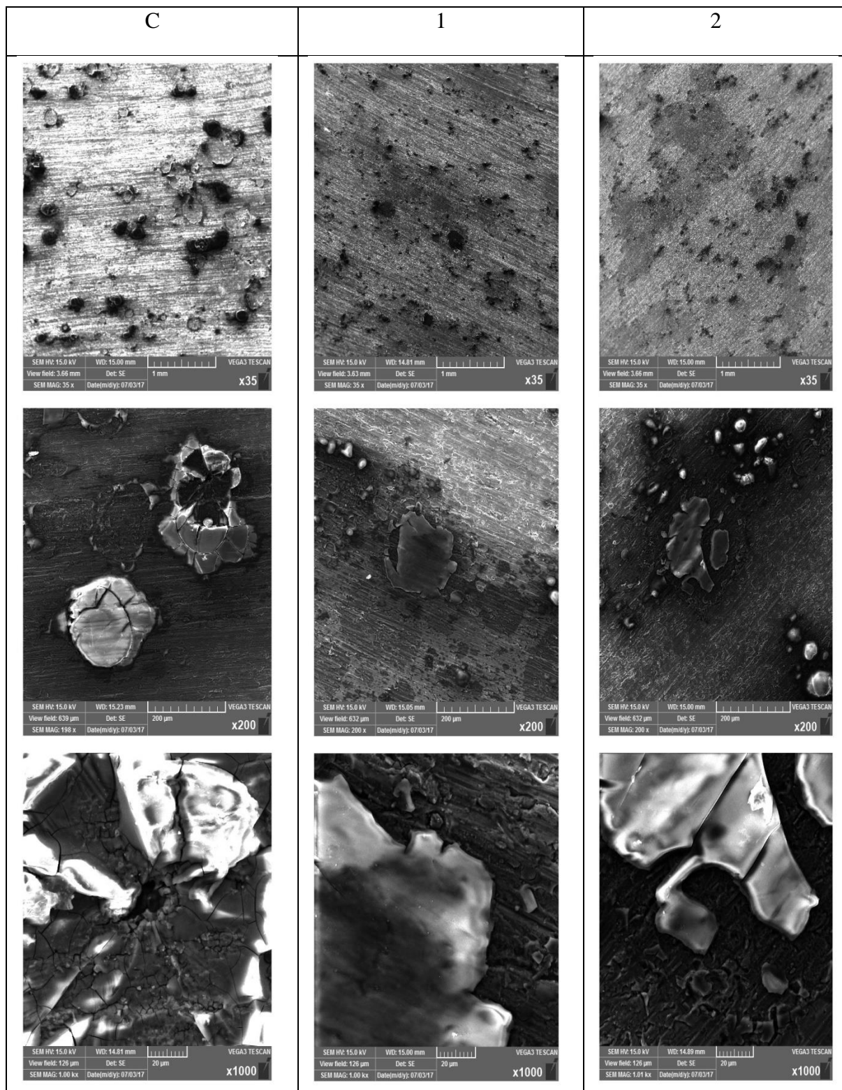
Tablica 13. Fotografije pločica nakon 10 dana izlaganja destiliranoj vodi u neinhibiranom sustavu (C), u sustavu s inhibitorom obloženim stijenka posude (1) i sustavu s otopljenim inhibitorom (2) snimljene elektronskim mikroskopom pri uvećanju 35 x, 200 x, 1000 x.
