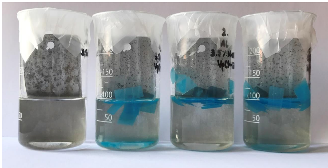
Slika 28. Nasoljene pločice u 3,5% otopini NaCl-a s različitim koncentracijama otopljenog VCI i čistoj 3,5% otopini NaCl-a nakon 7 dana izlaganja.
