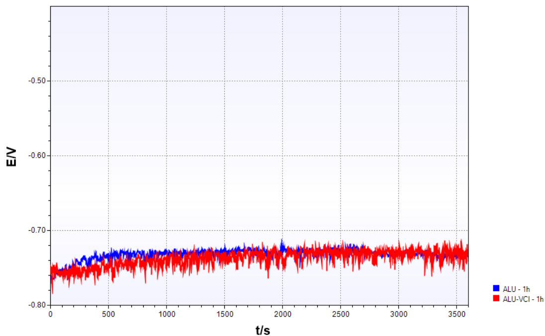
Slika 24. Vremenska ovisnost potencijala otvorenog kruga nakon izlaganja aluminijevih pločica inhibiranoj (VpCI) i neinhibiranoj 3,5% otopini NaCl-a.
