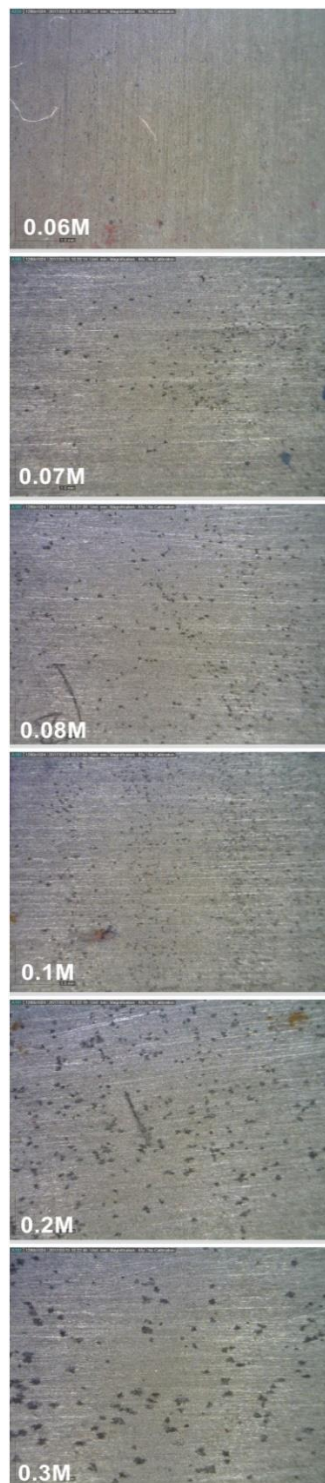
Slika 21. Testne površine nakon izlaganja bakrovim ionima (različitih koncentracija) snimljene svjetlosnim mikroskopom pod povećanjem 65 x.
