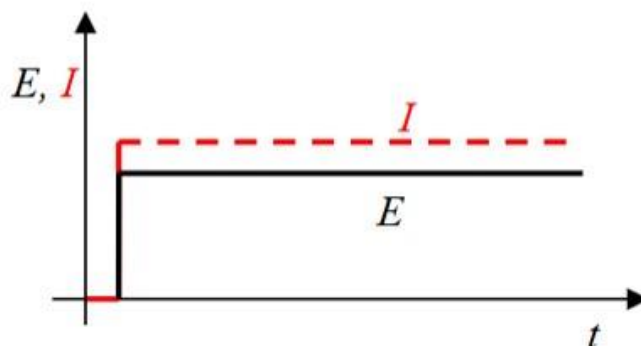
Slika 2. Narinuti potencijal i odziv struje u ovisnosti o vremenu u DC teoriji (kod f = 0 ) [14].
