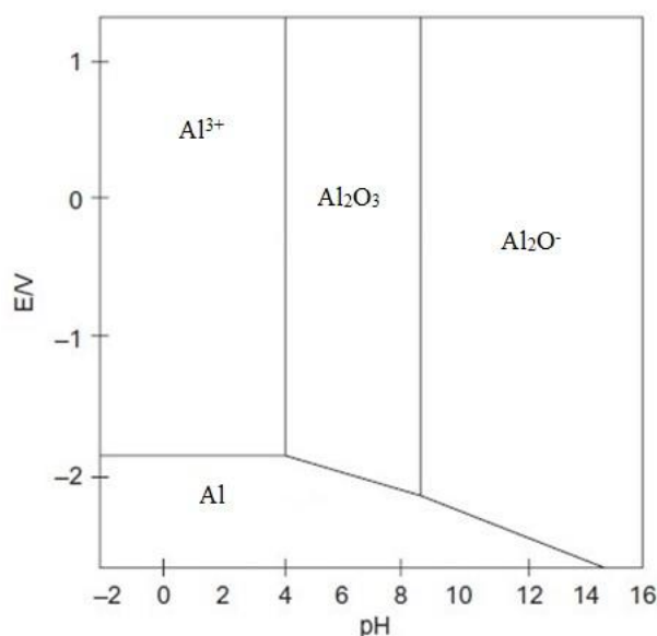
Slika 9. Pourbaixov dijagram aluminija u vodenim otopinama pri 25°C [16].
