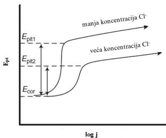
Slika 10. Shematski prikaz potencijala „pita“ na krivulji anodne polarizacije za aluminijeve legure [16]
