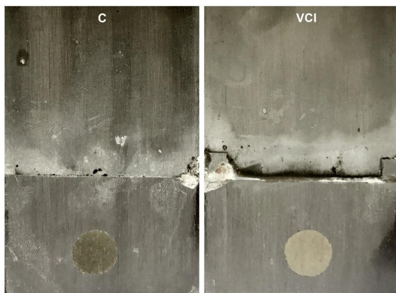
Slika 23. Testne površine nakon 60 dana izlaganja neinhibiranoj i inhibiranoj 3,5% otopini NaCl-a.
