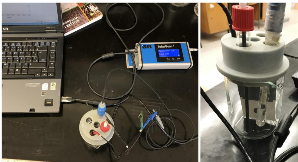
Slika 16. Aparatura za elektrokemijsko impedancijsko mjerenje.
