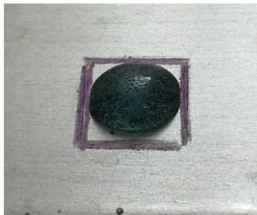
Slika 13. Izlučivanje bakra na aluminiju
