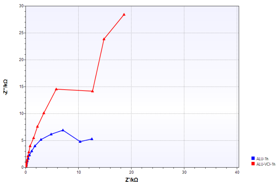
Slika 26. Nyquistov prikaz EIS spektra nakon 1h izlaganja aluminijskih pločica inhibiranoj (VCI) i neinhibiranoj 3,5% otopini NaCl-a
