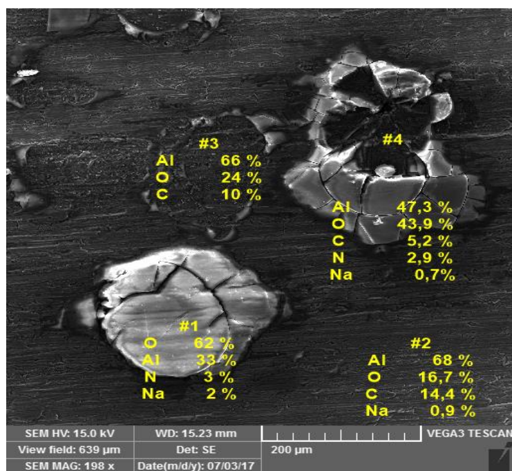
Slika 31. Analiza udjela elemenata na površini aluminijske pločice nakon 10 dana izlaganja destiliranoj vodi u neinhibiranom sustavu (C).
