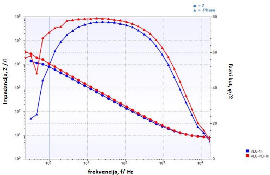
Slika 25. Bodeov prikaz EIS spektra nakon 1h izlaganja aluminijskih pločica inhibiranoj (VCI) i neinhibiranoj 3,5% otopini NaCl-a.
