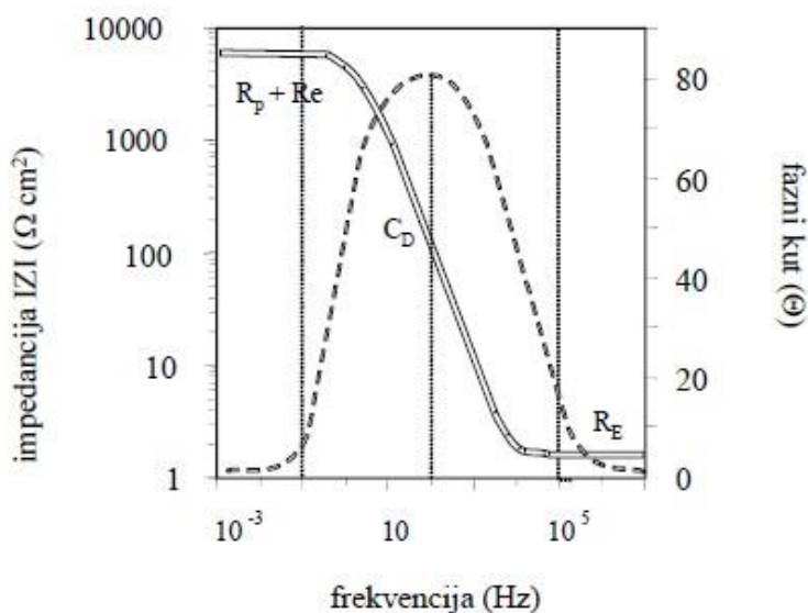
Slika 7. Bodeov dijagram za jednostavan elektrokemijski sustav [1].
