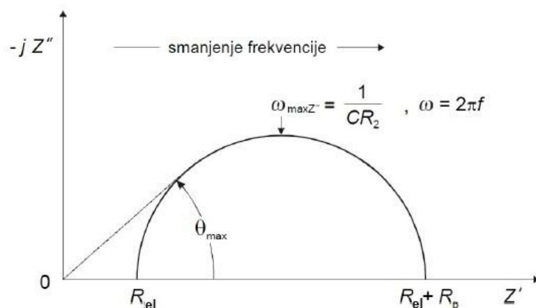
Slika 6. Nyquistov dijagram za jednostavan elektrokemijski sustav [13].
