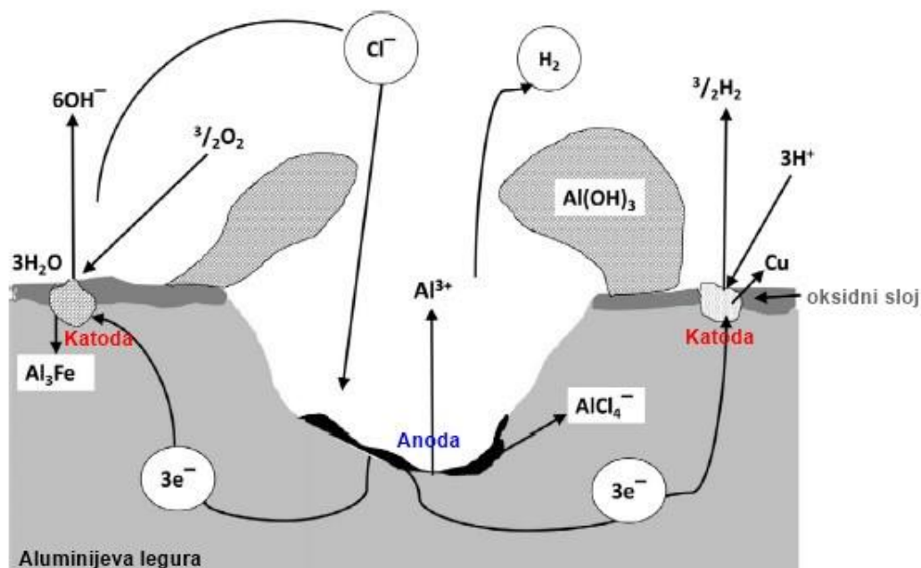
Slika 11. Shematski prikaz jamičaste korozije aluminijeve legure u kloridnoj otopini [19]
