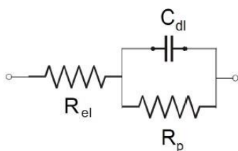
Slika 5. Randlesov krug jednostavne elektrokemijske ćelije [13].
