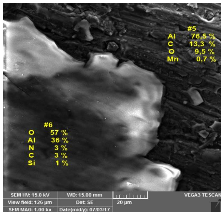
Slika 32. Analiza udjela elemenata na površini aluminijske pločice nakon 10 dana izlaganja destiliranoj vodi u sustavu s inhibitorom obloženim stjenkama posude (1).
