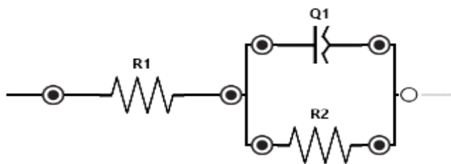
Slika 17. Ekvivalentni krug za modeliranje podataka EIS metode.
