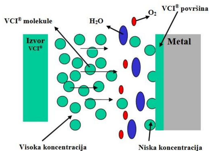
Slika 1. Mehanizam djelovanja parnofaznog inhibitora [5].
