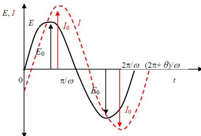
Slika 3. Narinuti potencijal i odziv struje u ovisnosti o vremenu u AC teoriji (kod f \neq 0 ) [14].
