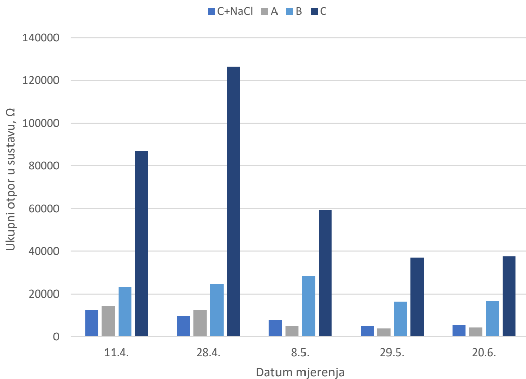
Slika 27. Grafički prikaz promjene ukupnog otpora u vremenu za ispitivane uzorke
