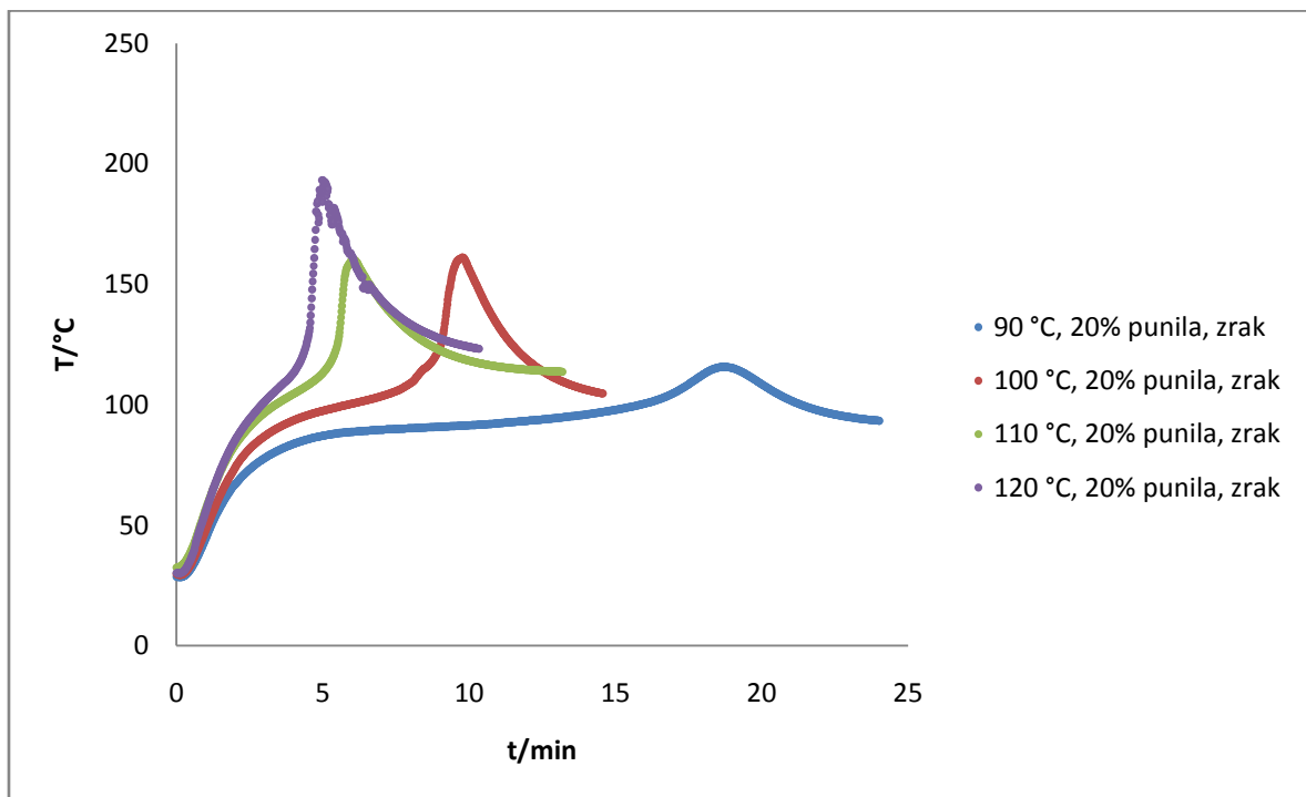
Slika 15. Ovisnost temperatura u centru malog kalupa pri različitim temperaturama zračne kupelji na protoku od 36\text{ l/min} s dodatkom 20% punila s 1% TBPB inicijatora.
