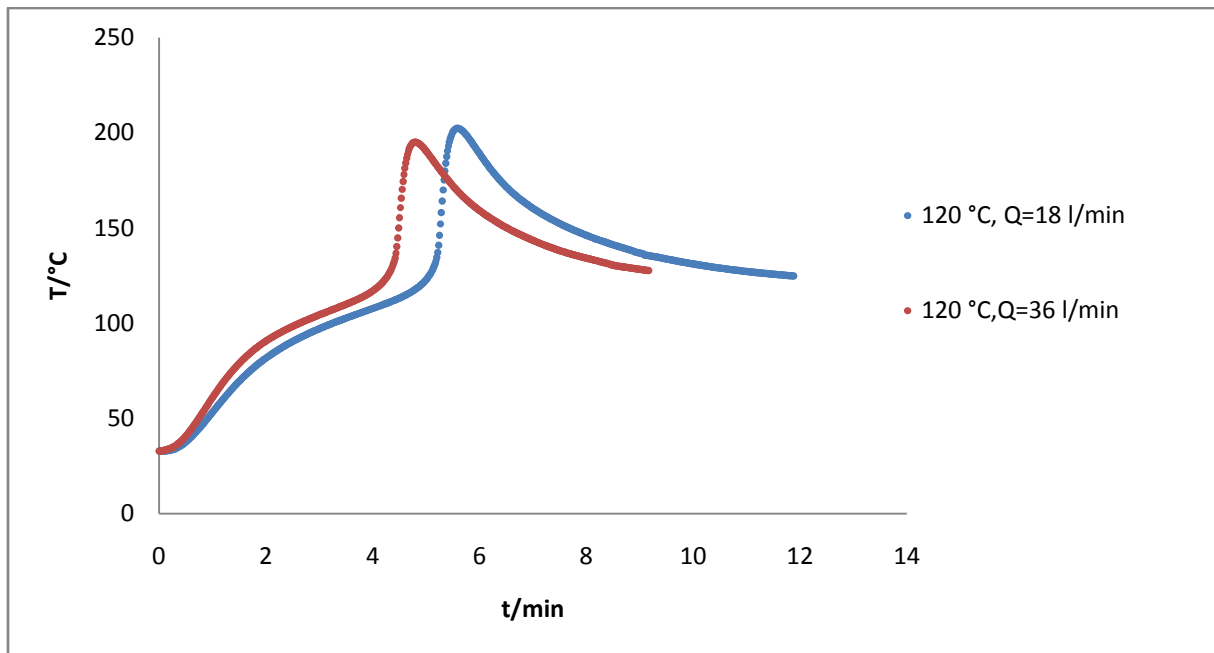
Slika 14. Grafički prikaz utjecaja protoka zraka u zračnoj kupelji na očvršćivanje smole s 1% TBPB inicijatora u malom kalupu pri 120^\circ\text{C} .
