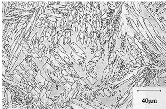
Slika 2. 4. Mikrostruktura dupleks čelika
