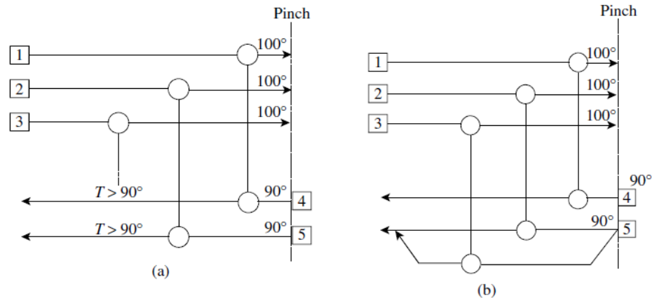
Slika 2.11. Dijeljenje struja iznad pincha
