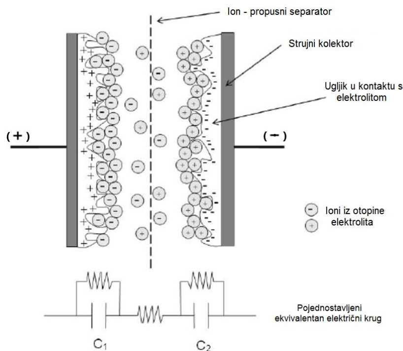
Slika 5. Shematski prikaz elektrokemijskog dvoslojnog kondenzatora [15]
