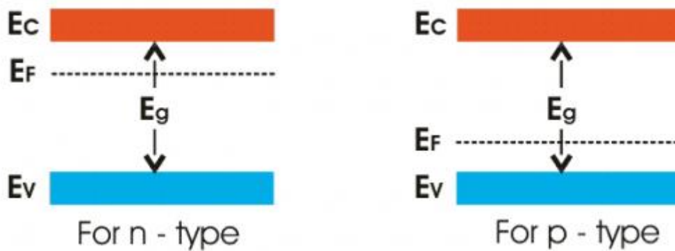
Slika 5. Dijagrami energetske vrpce za ekstrinzične poluvodiče
