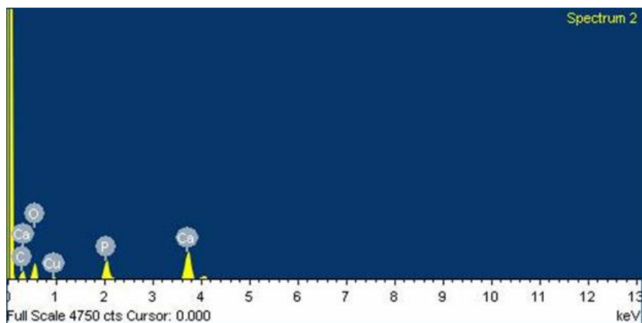
Slika 5.8. EDS spektar površine uzorka čestica kalcijevog karbonata sintetiziranih pri T = 40\text{ }^{\circ}\text{C} uz koncentraciju enzima c (ureaza) = 2\text{ mg mL}^{-1} (eksperiment 5).
