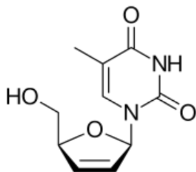
stavudin
