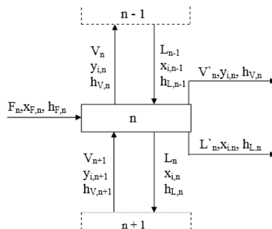
Slika 9. Ravnotežni stupanj jedne teorijske plitice
